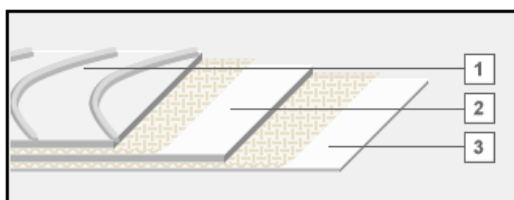
Type X Bogenprofil groß
