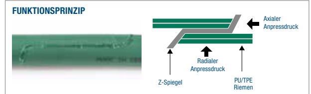
Kompakte Führungseinheit für Überlappverschweißungen mittels Z-Spiegel mit radialem und axialem Anpressdruck.
